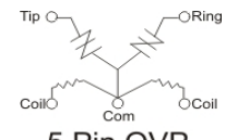
5 Pin OVP
